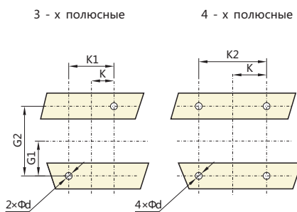
Разметка шин
