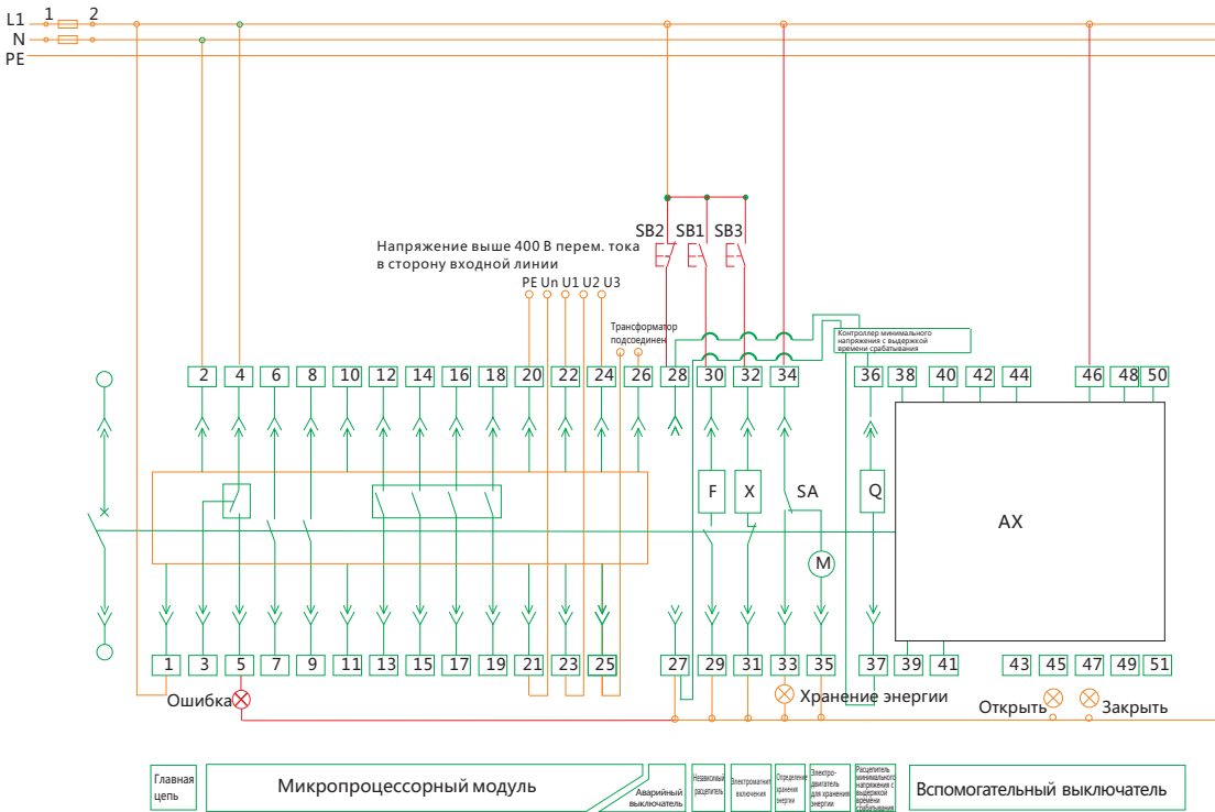
Вторичная схема микропроцессорного блока типа 3М NA1-2000X~6300X (с распрепителем минимального напряжения с задержкой)
