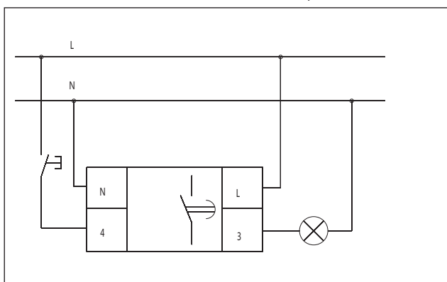
Рис. 3, электрическая схема NJS3-A
