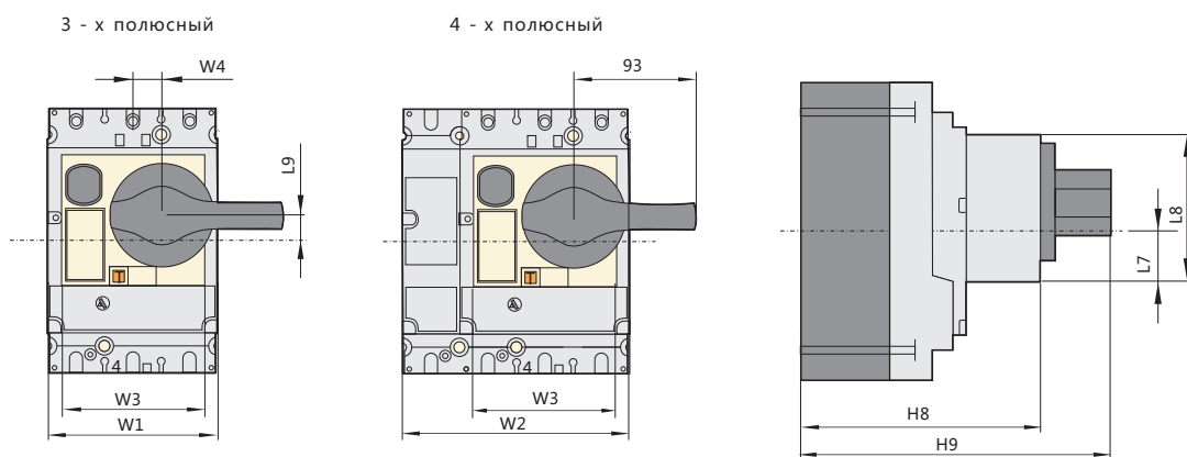
Разметка панели ( для выключателей стационарного и втычного исполнения)
