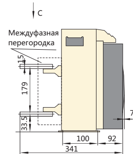
Горизонтальное присоединение
