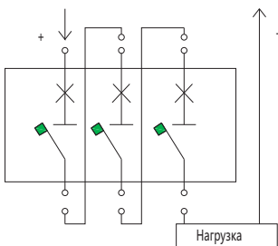
Схема С: Использование трёх полюсов для разрыва цепи одной полярности .
