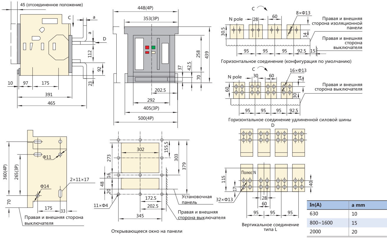
Выключатель выдвижного типа вертикальный, заднее подсоединение NA1-2000X/NA1-2000XN/NA1-2000XH
