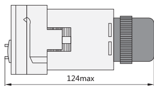
Профильные установочные размеры
