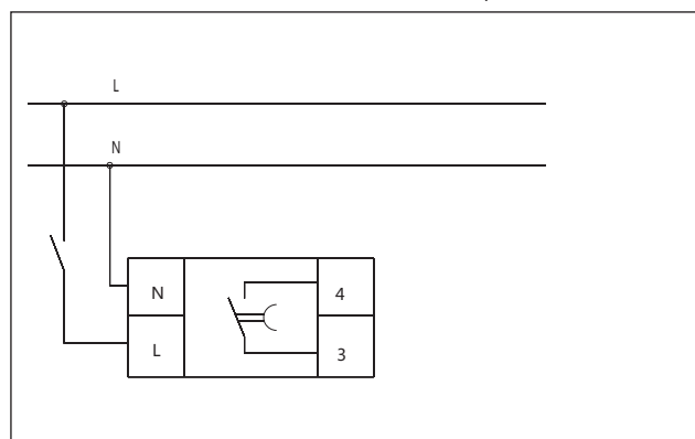
Рис. 4, электрическая схема NJS3-B
