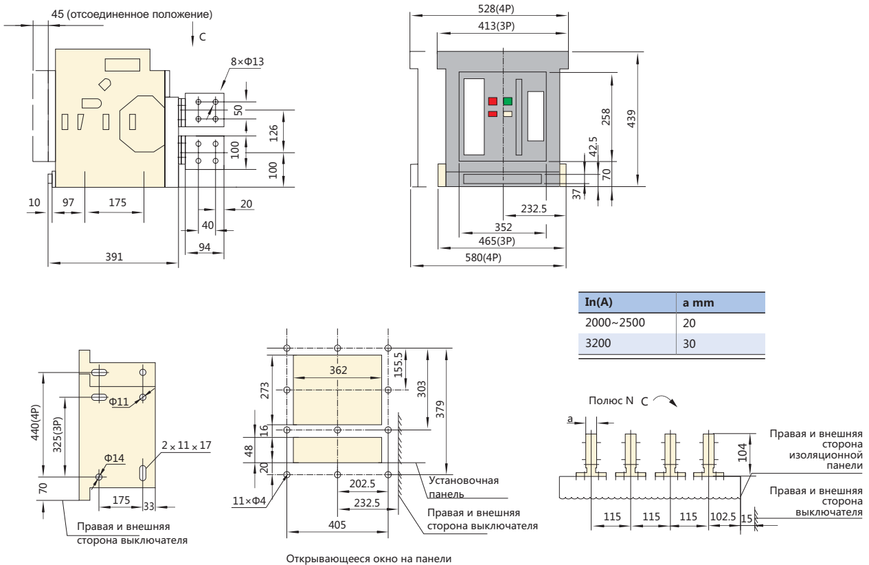
Выключатель выдвижного типа горизонтальный, заднее подсоединение NA1-3200X/NA1-3200XN
