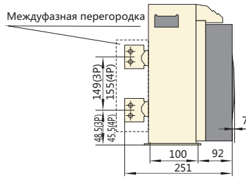
Вертикальное присоединение
