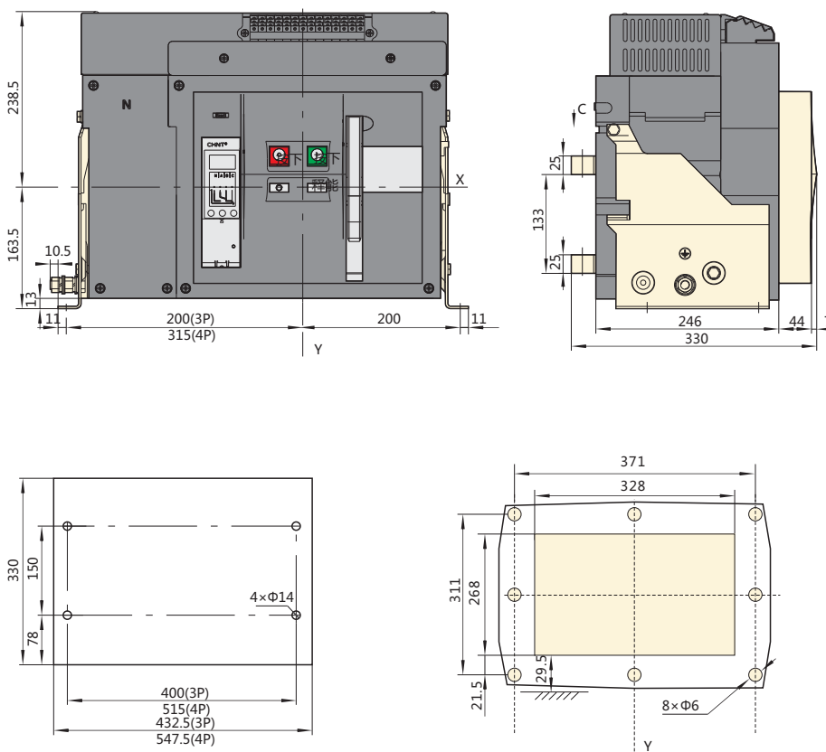
NA8G-4000 стационарное исполнение, заднее присоединение, горизонтальные контактные пластины
