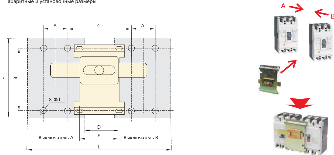
Габаритные и установочные размеры
