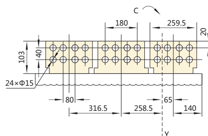
NA8G-6300(I n =6300A) выдвижное исполнение, заднее присоединение, горизонтальные контактные пластины
