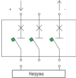
Схема А: Использование по одному полюсу для разрыва цепи каждой полярности
