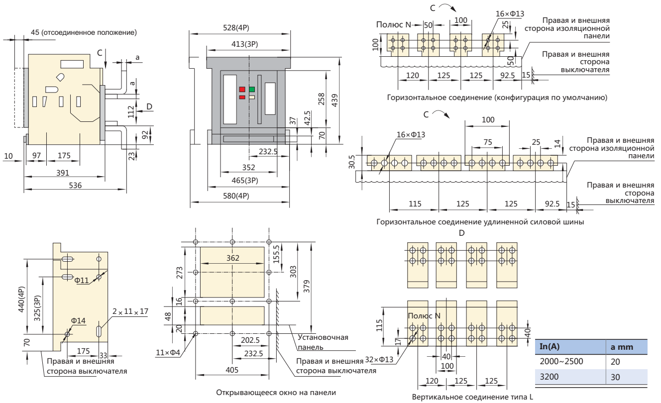
Выключатель выдвижного типа NA1-3200X/NA1-3200XN
