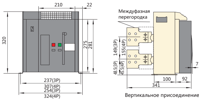
Вертикальное присоединение
