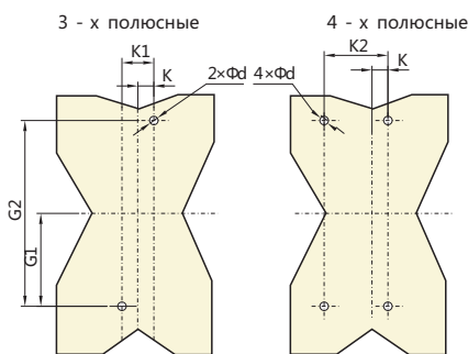
Разметка монтажной панели
