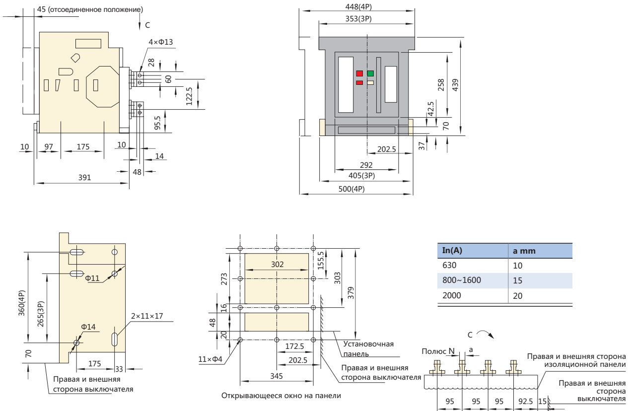
Выключатель выдвижного типа вертикальный, заднее подсоединение NA1-2000X/NA1-2000XN/NA1-2000XH
