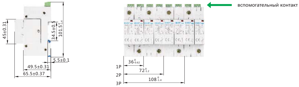
Габаритные и установочные размеры NU6-II/F (40 кА) без вывода для дистанционного управления
